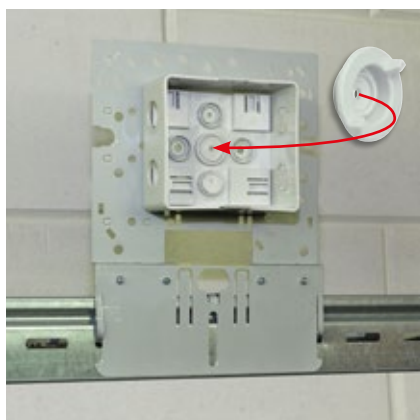
Montageplaatbevestiging
